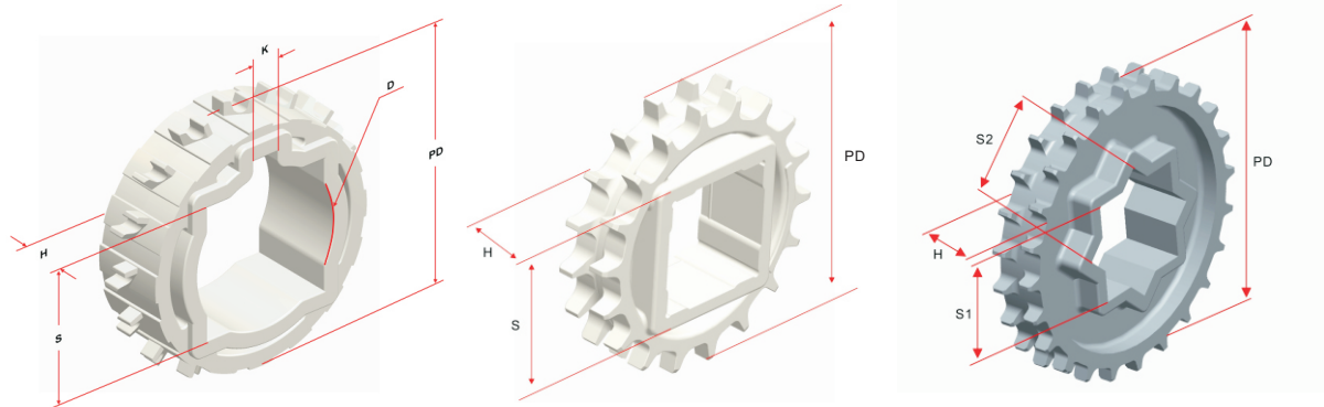
Sprocket Dimensions
