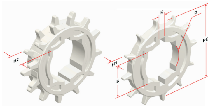
Sprocket Dimensions
